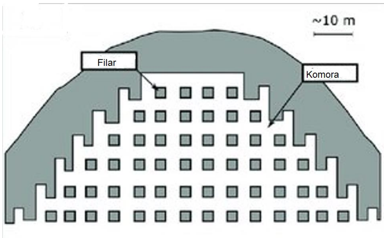
Rys.5. Komorowo-filarowy system wybierania węgla.
