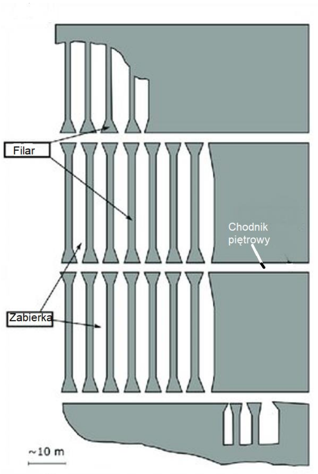
Rys.6. Brytyjski system wybierania węgla długimi zabierkami tzw. Bord & Pillar.
