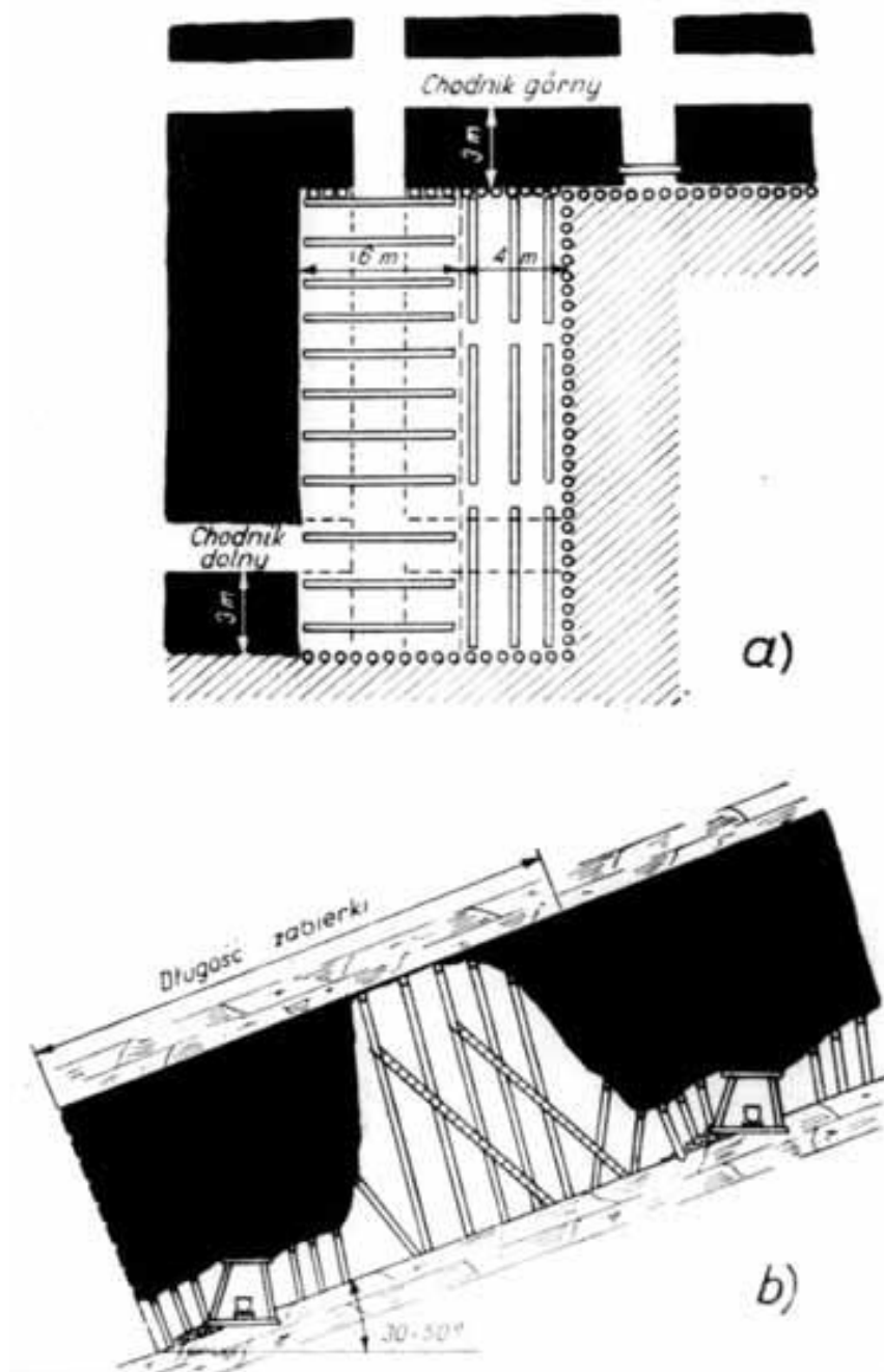
Rys. 17. System zabierkowy wybierania grubego pokładu w kopalni Ferdinand (Katowice).
