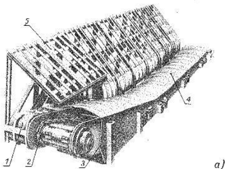
Rys. 23. Samoładujący przenośnik zabierkowy ROK-60.
