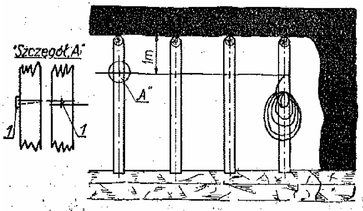
Rys. 12. Zabezpieczanie stojaków drewnianych przed w zabierce.
