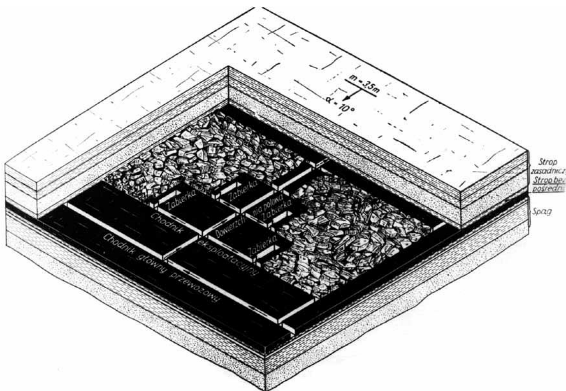
Rys.18. Schemat rozcinki dla wysokich zabierek w kop. Ferdynand (Katowice).
